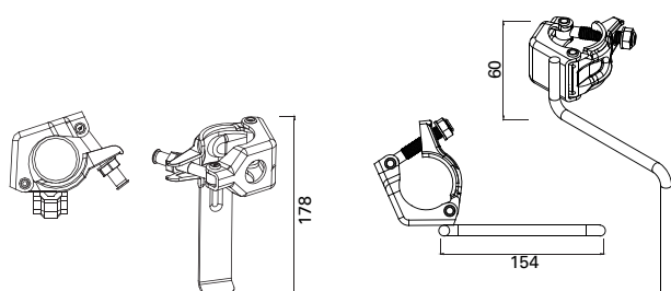
アルスピーダー 専用ホルダー
