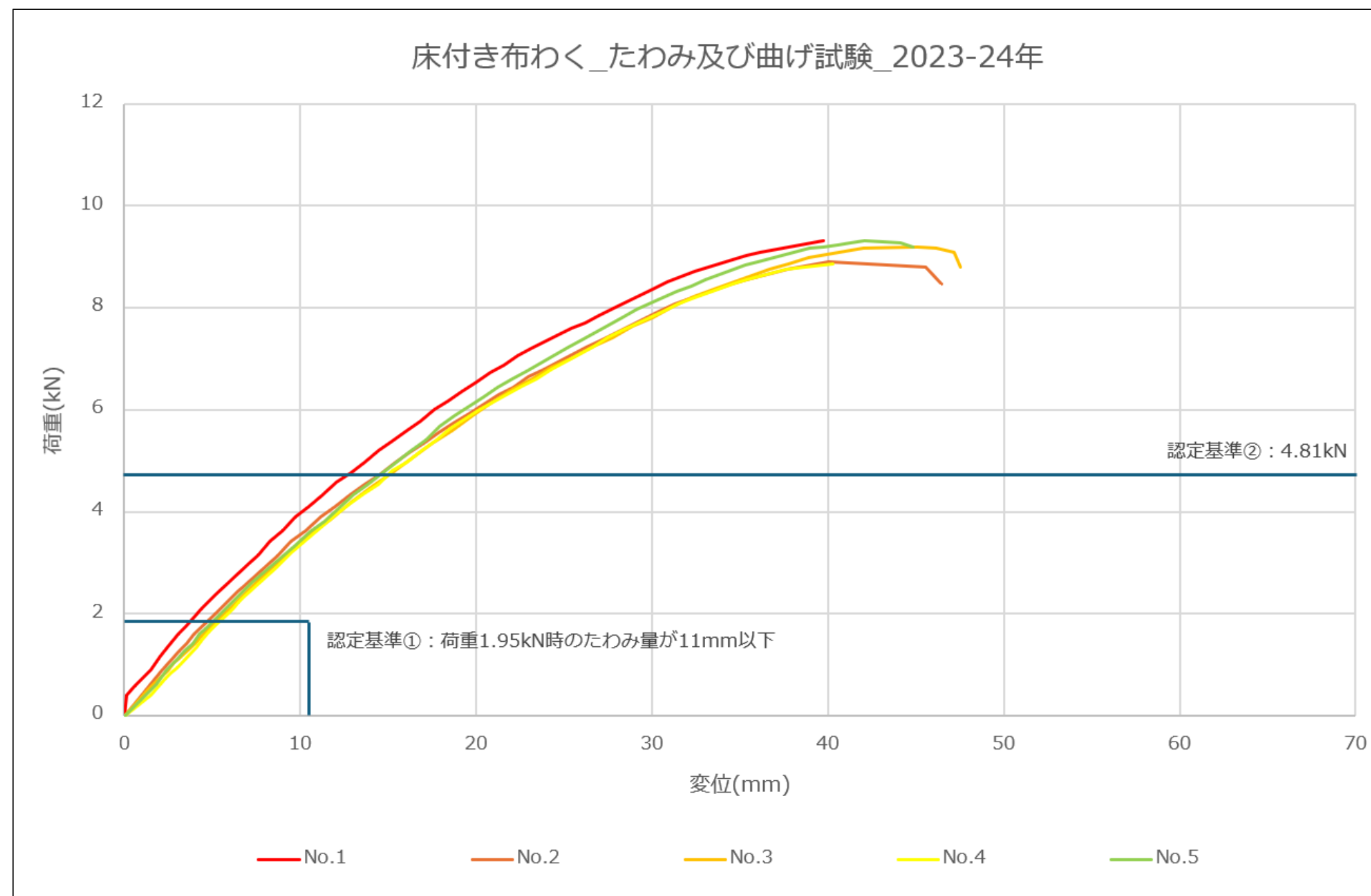
床付き布わく_たわみ及び曲げ試験_2023,24年の折れ線グラフ
