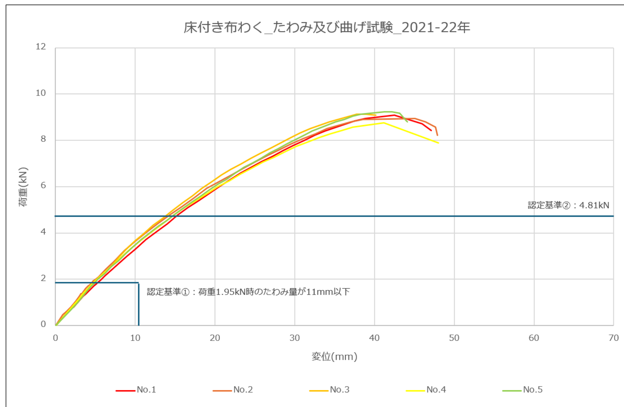
床付き布わく_たわみ及び曲げ試験_2021,22年の折れ線グラフ
