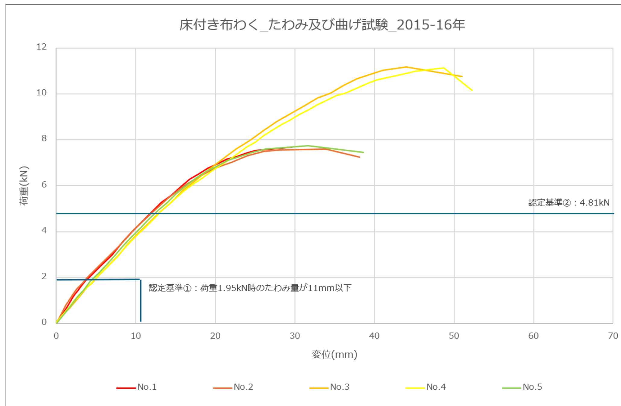
床付き布わく_たわみ及び曲げ試験_2015,16年の折れ線グラフ
