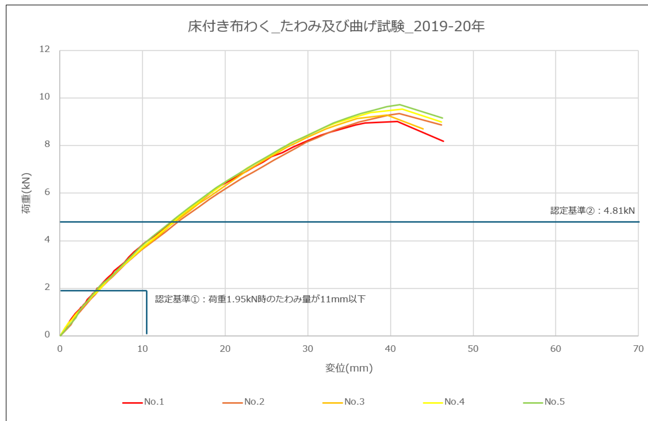
床付き布わく_たわみ及び曲げ試験_2019,20年の折れ線グラフ
