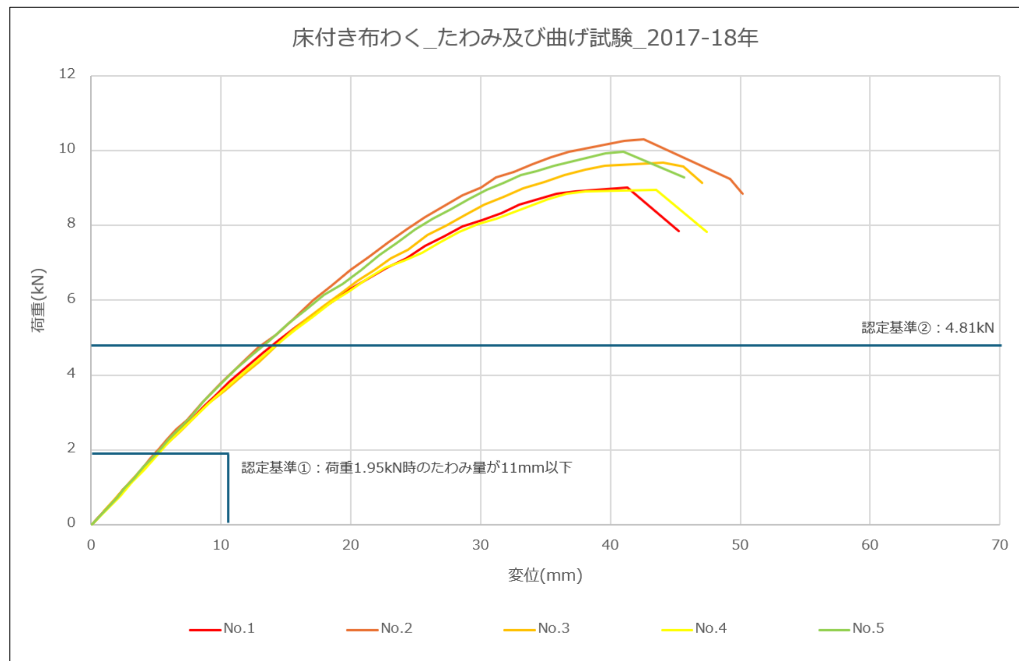
床付き布わく_たわみ及び曲げ試験_2017,18年の折れ線グラフ
